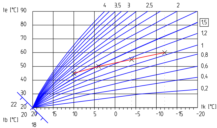
Vaillant CalorMatic szabályzó szabályozási görbék
