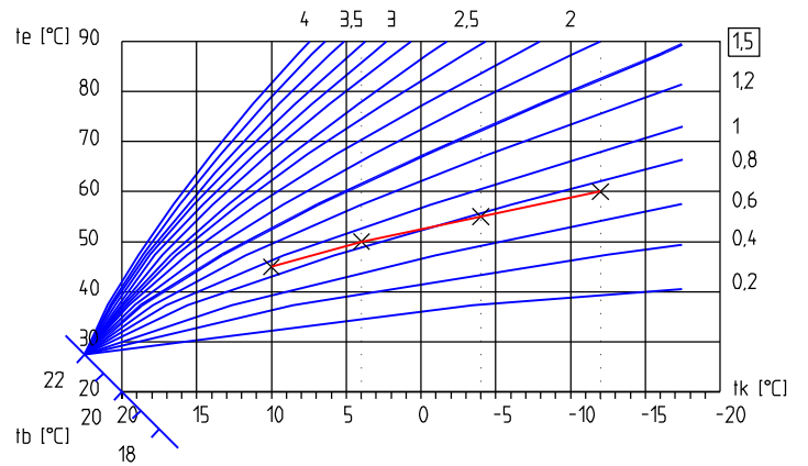
Vaillant CalorMatic szabályzó szabályozási görbék
